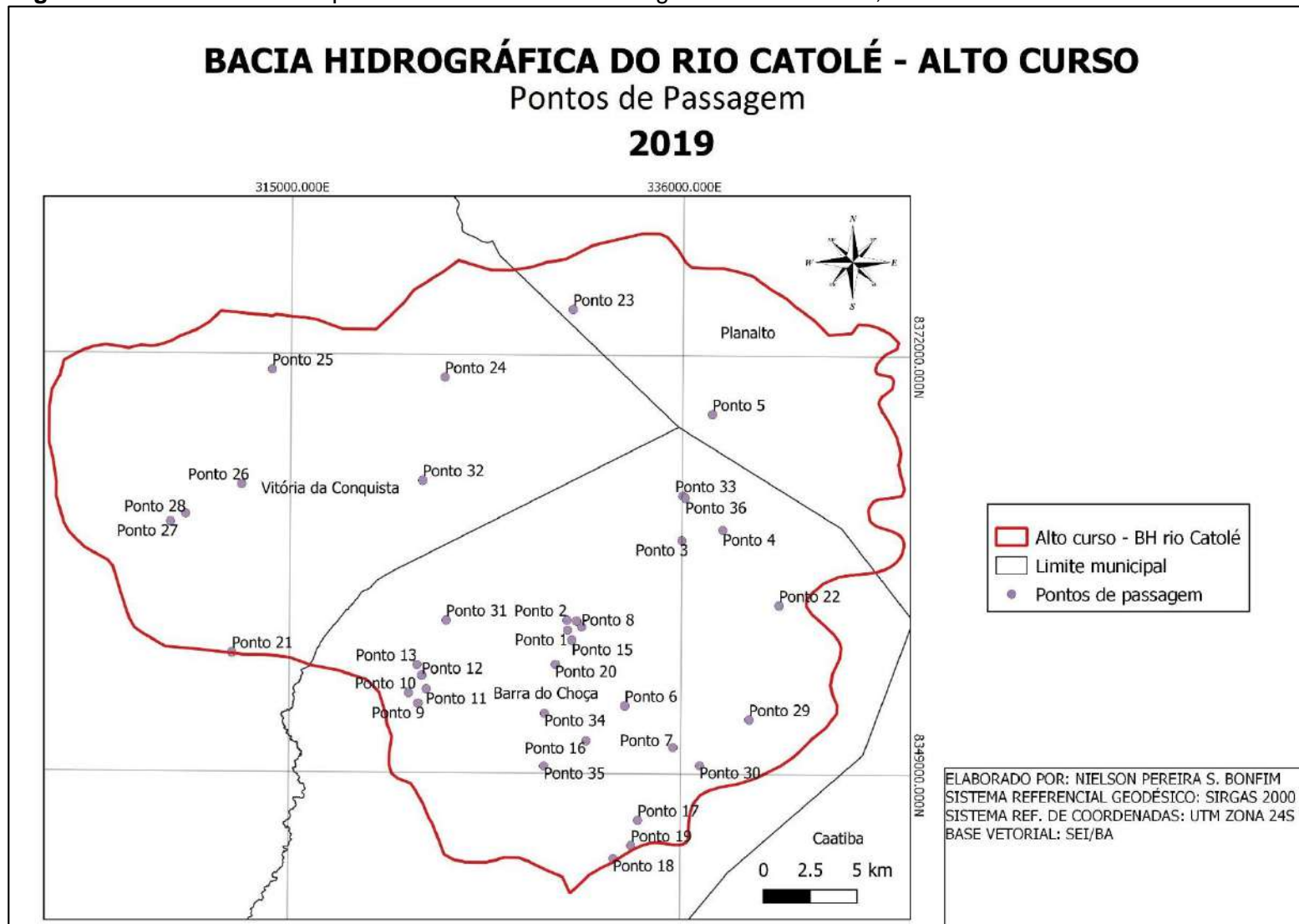
Figura 18 – Trabalho de campo – Alto curso da bacia hidrográfica do rio Catolé, 2019.
