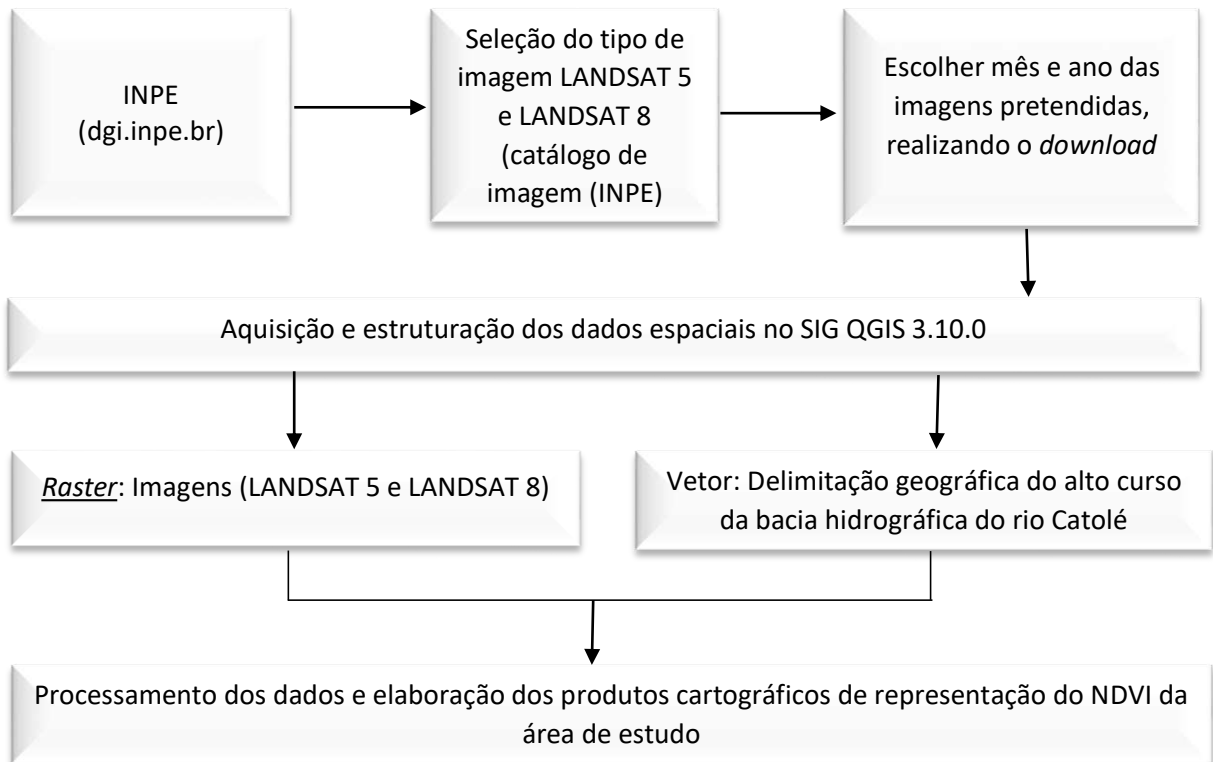
Figura 4 – Fluxograma da metodologia de NDVI e SAVI.
