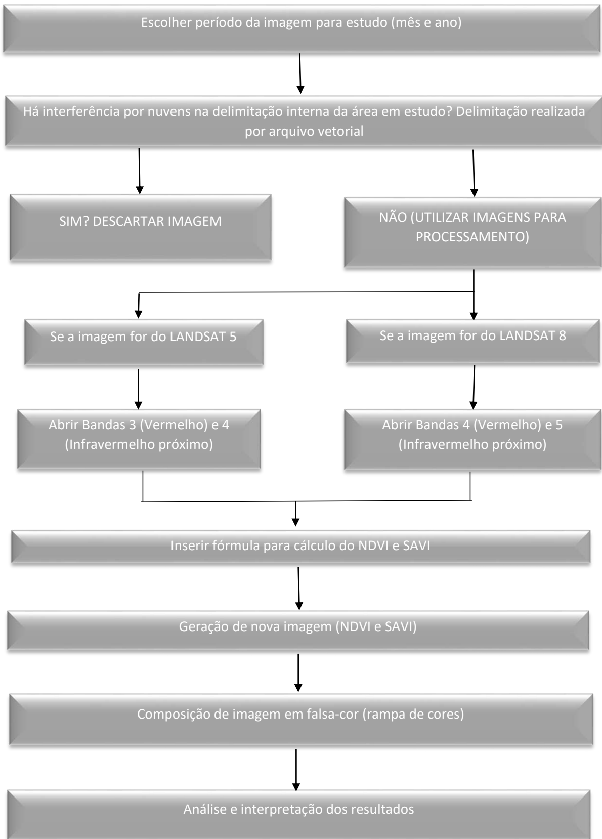
Figura 5 – Fluxograma de processamento das imagens – LANDSAT 5 e 8.
