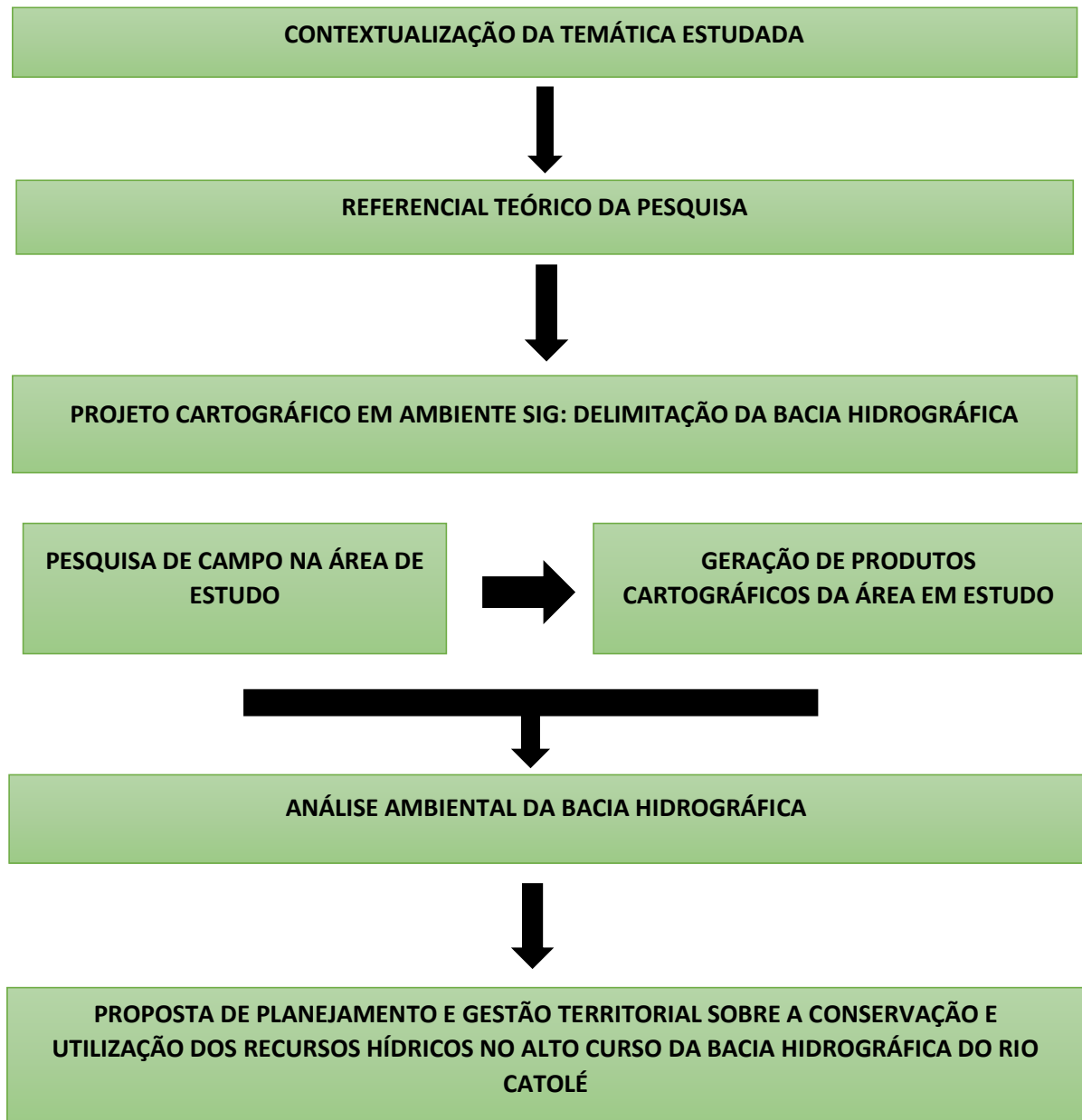
Figura 2 – Fluxograma do procedimento metodológico da pesquisa.
